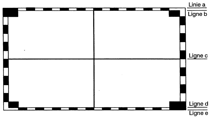
Fig. 5 Croix centrale, 625 / 525 lignes, format d'image 16:9
