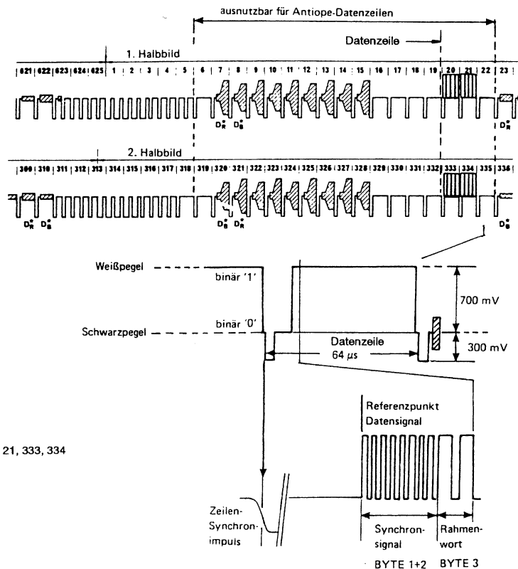
Fig. 3 Lage und Pegel von Antiope-Datenzeilen
