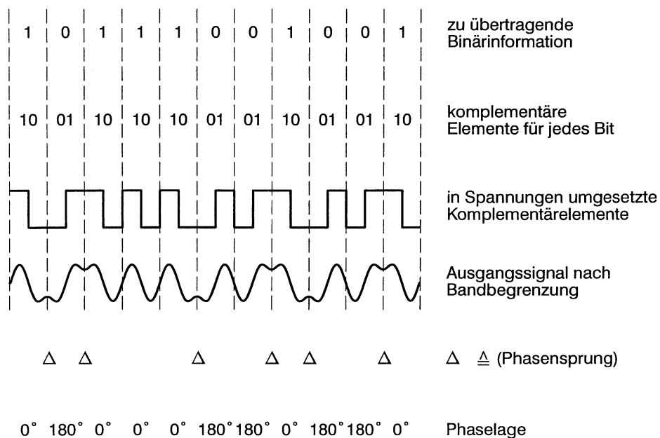
Fig. 6 Erzeugung des Biphas-Code
